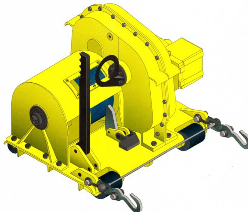
Bulldog Winch Model 41750-3-41BG NSN 1680-00-860-3934LG
